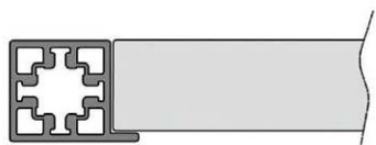
Профиль для вставной панели 16 мм толщиной
